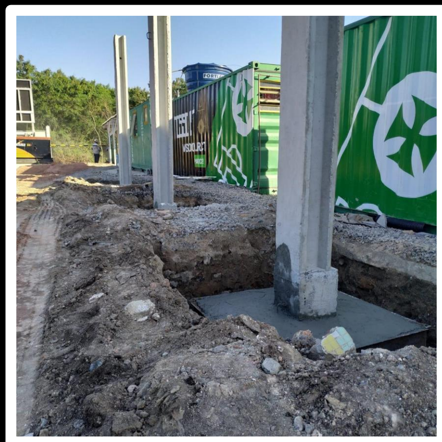
CONCRETAGEM DAS SAPATAS DO MURO DA LATERAL DIREITA
